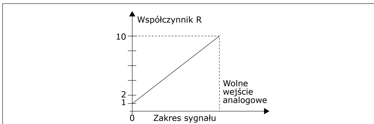
Rys. 52: Zmniejszenie czasów przyspieszania i hamowania
