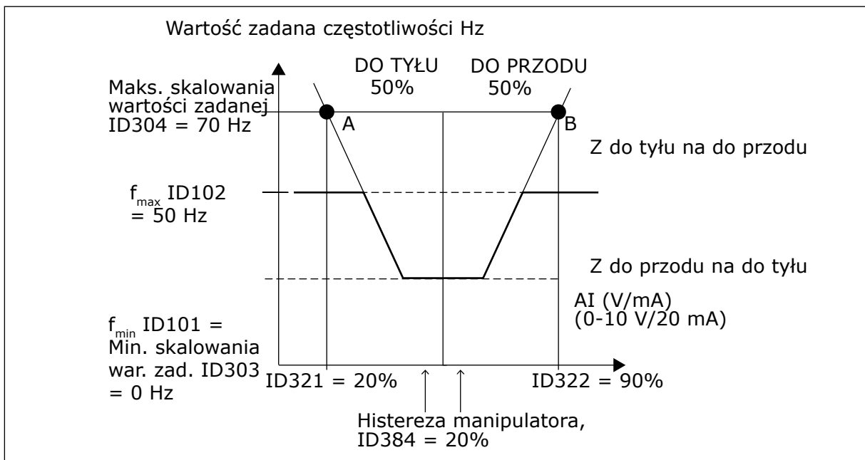
Rys. 60: Hystereza manipulatora z częstotliwością minimalną 35 Hz
